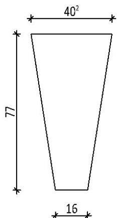
VB077 keresztmetszet
