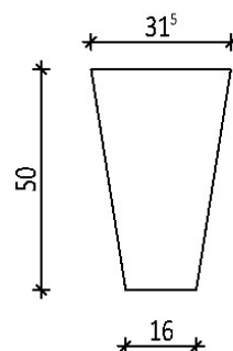
VB050 keresztmetszet
