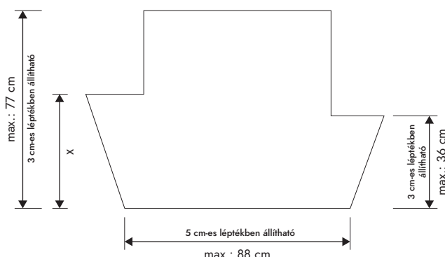
DB gerenda keresztmetszet Aszimmetrikus fülgeometria
