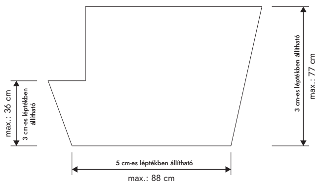
LB gerenda keresztmetszet - Egyéb verzió
