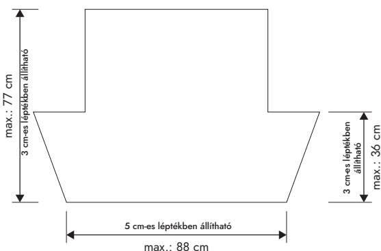
DB gerenda keresztmetszet Szimmetrikus fülgeometria
