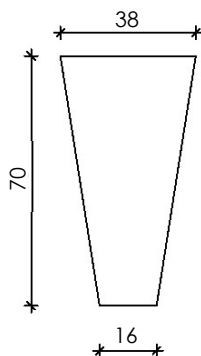
VB070 keresztmetszet
