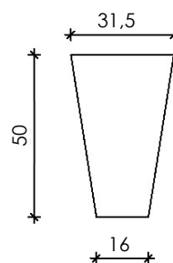
VB050 keresztmetszet
