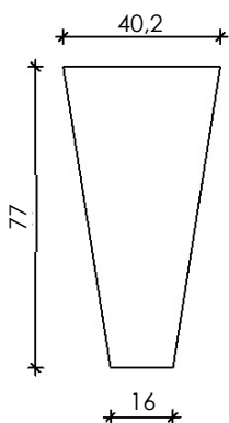
VB077 keresztmetszet
