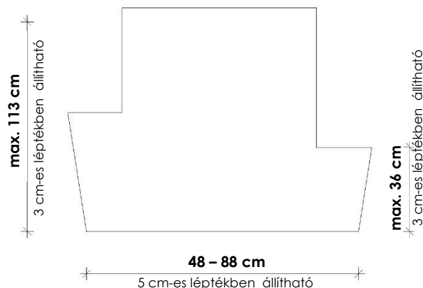
DB gerenda keresztmetszet Aszimmetrikus fülgeometria
