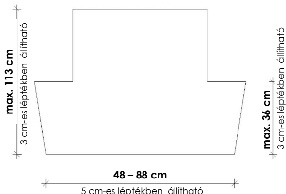
DB gerenda keresztmetszet Szimmetrikus fülgeometria
