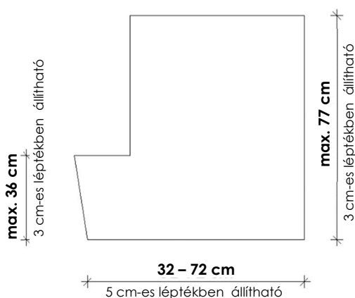
LB gerenda keresztmetszet
